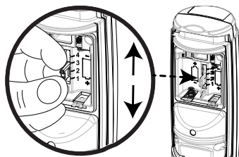
Figure 32. Sélecteur de non déclenchement par les animaux
