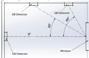
Figura 3. Ángulo entre detector y ventana
