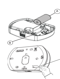
Figure 5. Vue intérieure
