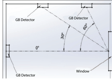
Figure 3. Angle entre la fenêtre et le détecteur
