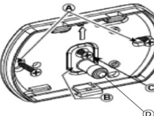
Figura 7. Vista interna del PGx922
