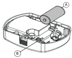
Figura 6. Inserção da bateria
