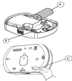
Figura 5. Vista interior
