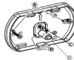
Figura 7. PG922 Vista interna
